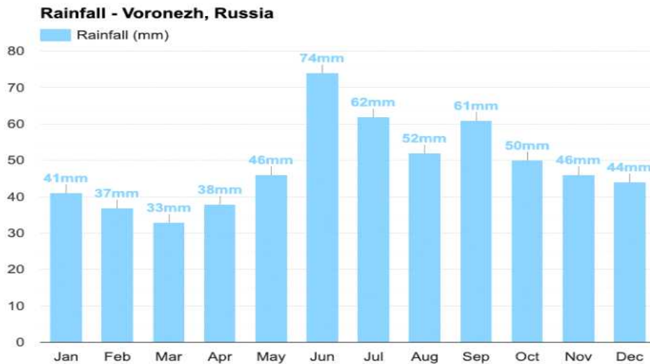
[그림 4. 보로네시주 강수량]
