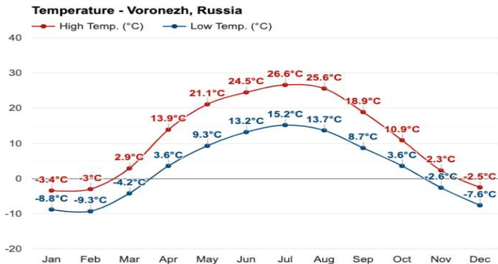
[그림 3. 보로네시주 기후 변화]
